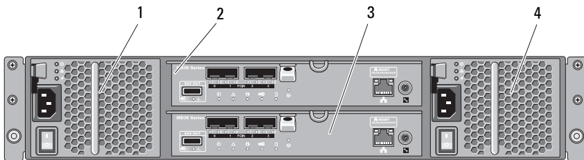
图 2-4. 背面板部件和指示灯—Dell PowerVault MD3600f 系列
